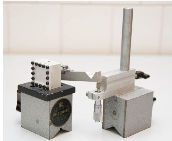
4. ábra. (a) A mérés eszközkészlete, (b) a deformálható membrán és a mozgatókar.
