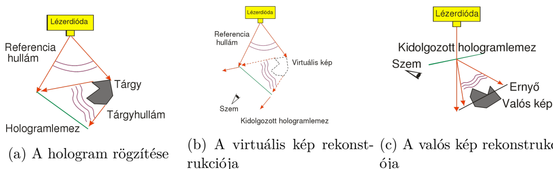
1. ábra. Transzmissziós off-axis hologram
