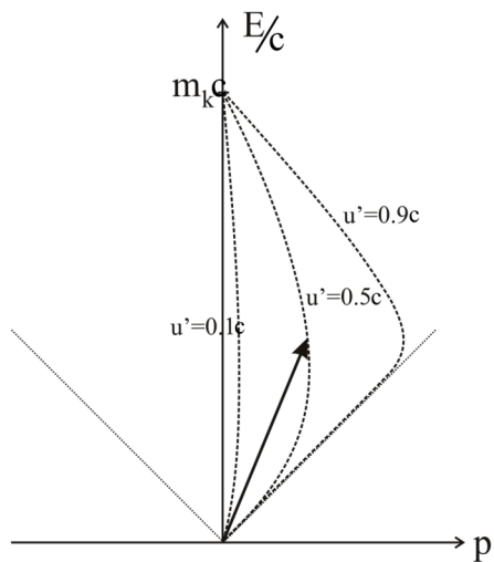
Relativisztikus rakéta 3. Rakéta-tömeg-görbék különböző hajtómű-sebességekre
