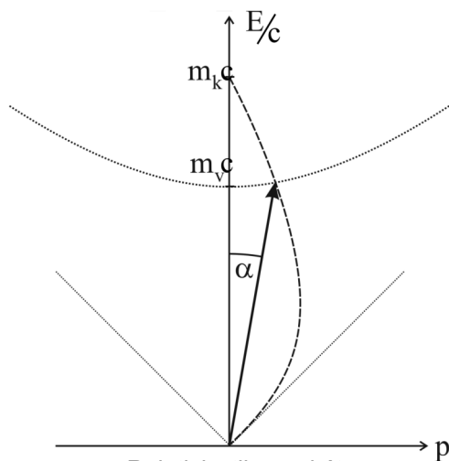
Relativisztikus rakéta 4. A végsebesség megállapítása grafikusán, adott kezdeti és végső tömegre.
