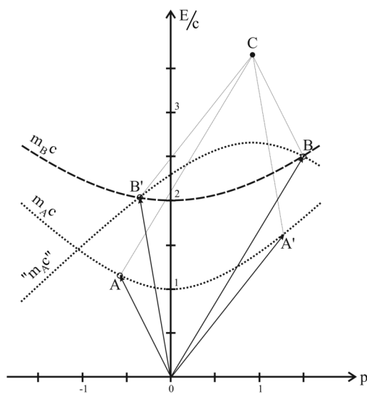
Rugalmas ütközés 1D-ben.
