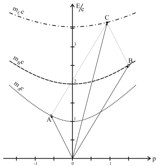
Rugalmatlan ütközés 1D-ben.
