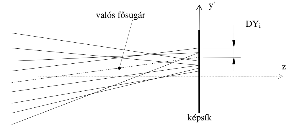
59. ábra. Egyetlen tárgypontból indított valós sugarak metszik a képsíkot.
