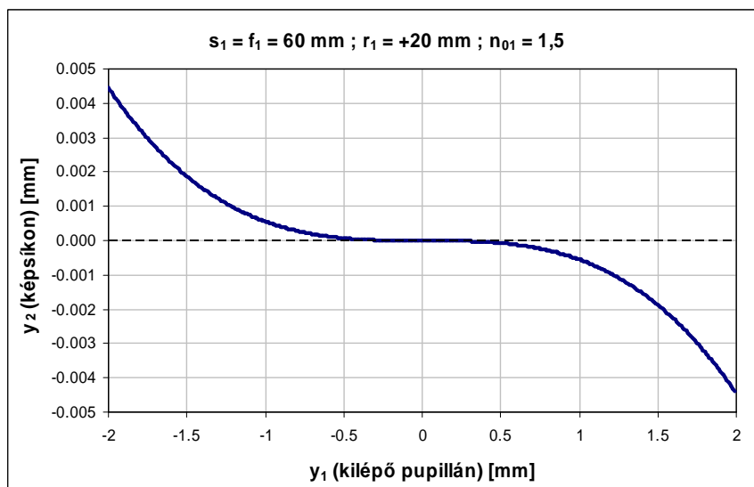
33. ábra. Nyíláshiba transzverzális hibagörbéje, a képsík paraxiális képsíkon.
