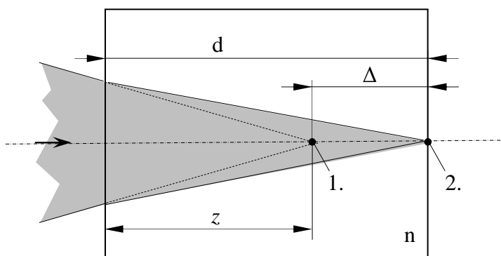
17. ábra. Anyagba fókuszált fénynyaláb pozíciójának megváltozása levegőbe fókuszált nyaláb esetéhez képest.
