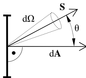
60. ábra. Sugársűrűség: egységnyi térszögbe eső Poynting-vektor mennyiség.
