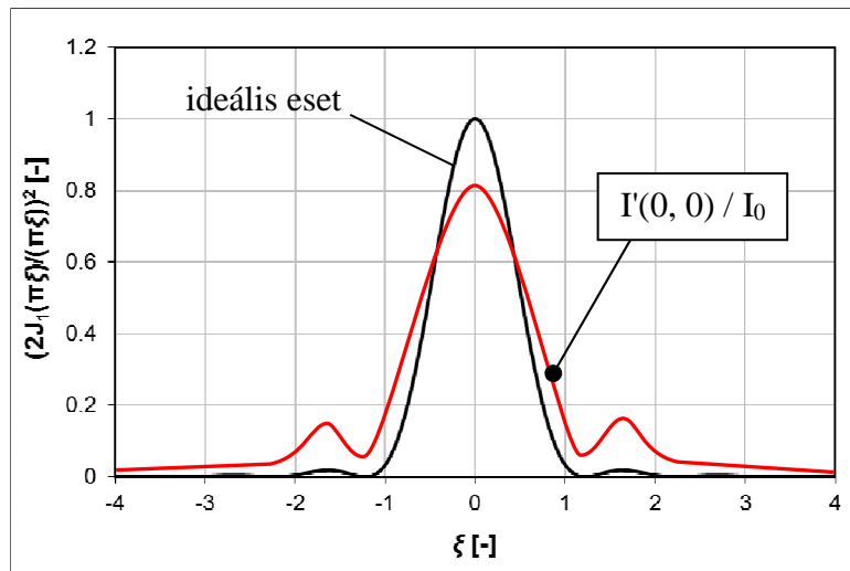
68. ábra. Kör alakú apertúra Fraunhofer-diffrakciós képe (intenzitás eloszlása), ideális hullámfront ( \text{RMS OPD} = 0 ) és aberrált hullámfront esetén ( \text{RMS OPD} > 0 ).
