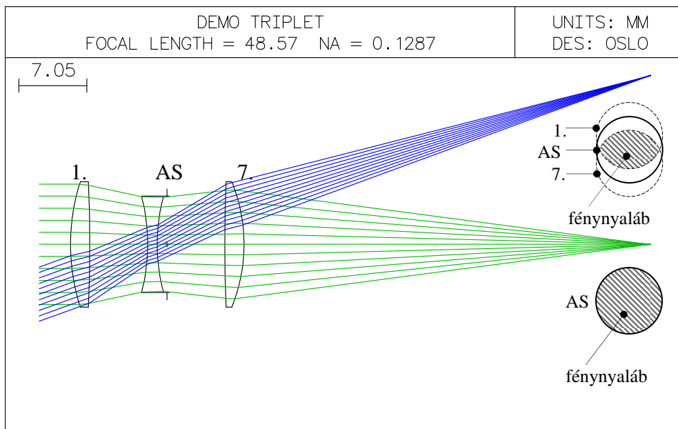
58. ábra. A vinyettálás szemléltetése.
