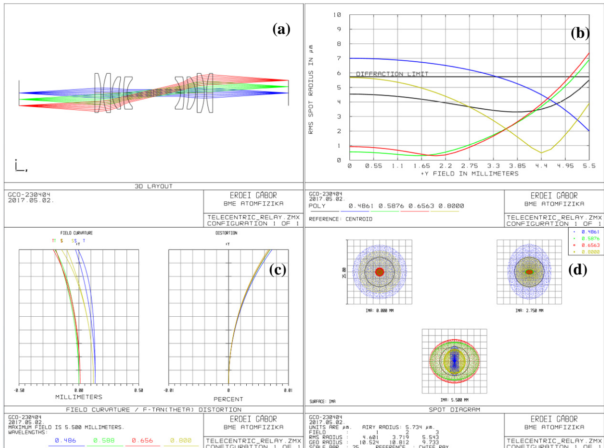
109. ábra. Telecentrikus képátvetítő objektív képe (a), a szóródási folt tárgyszög-függése (b), képmezőhajlás és torzítás (c), polikromatikus szóródási foltok három jellemző tárgypont esetén, ahol a körök az Airy-foltot szimbolizálják (d).
