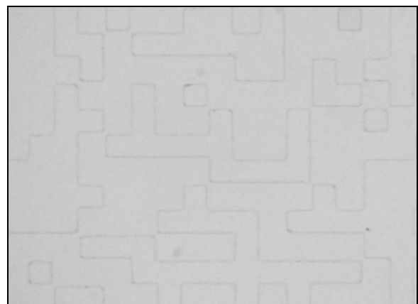
3. ábra. Fázistárgy leképzése térben inkohereus fényvel. A fázislépcsők határán fellépő destruktív interferencia láthatósága jelentősen romlott.
