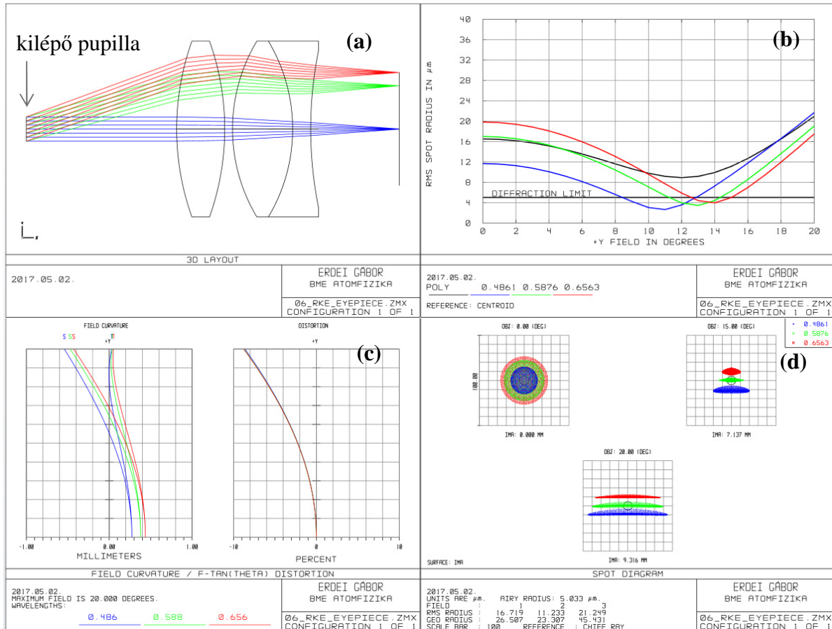
107. ábra. Mikroszkópeakulár képe (a), a szóródási folt tárgyszög-függése (b), képmezőhajlás és torzítás (c), polikromatikus szóródási foltok három jellemző tárgypontra esetén, ahol a körök az Airy-foltot szimbolizálják (d).
