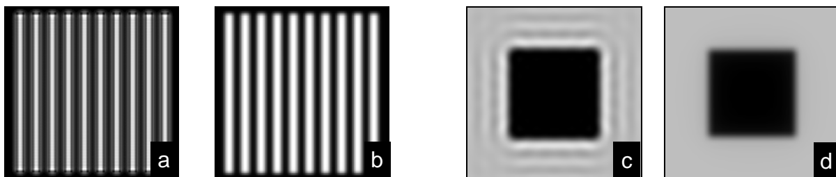
5. ábra. Amplitudótárgy (fekete-fehér négyzög rács) leképezése térben koherens (a) és inkoherens fénnel (b) . Koherens megvilágítás esetén a határokon diffrakciós csíkok jelennek meg. Inkoherens esetben a kapott kép kb. szinuszos besugárzás eloszlású.
