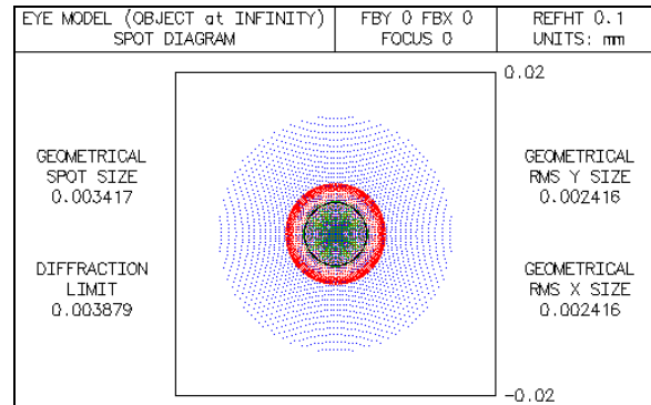
94. ábra. A szem szóródási foltja a retinán \varnothing 3 mm-es pupilla esetén. A kék szín defokuszáltságán jól látható a longitudinális színhiba.
