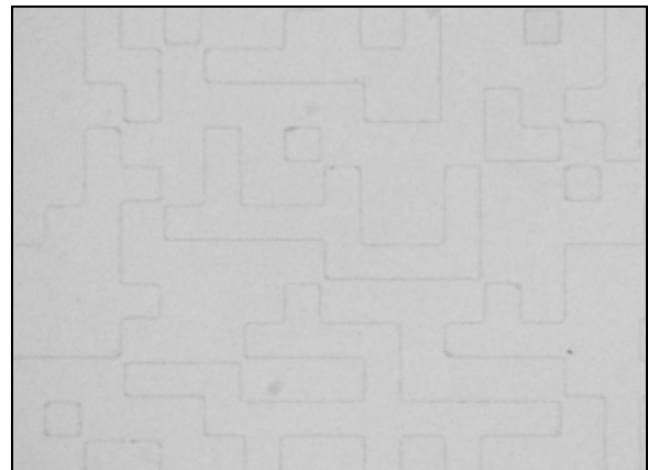
3. ábra. Fázistárgy leképzése térben inkoherens fényvel. A fázislépcsők határán fellépő destruktív interferencia láthatósága jelentősen romlott.
