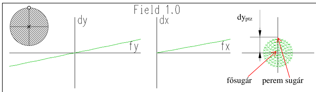
45. ábra. Petzvál-képzőhajlás hibagörbéje és szóródási foltja (ua. mint defókus). h \neq 0 .
