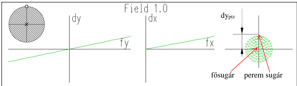
45. ábra. Petzvál-képzőhajlás hibagörbéje és szóródási foltja (ua. mint defókus). h \neq 0 .
