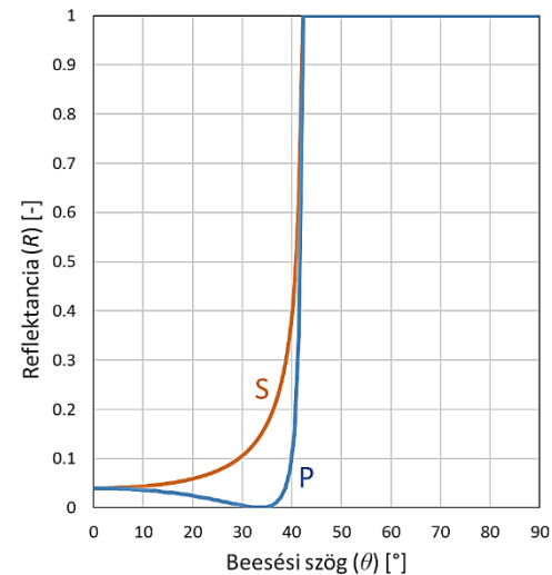
belső visszaverődés ( n/n' = 1.5 )
