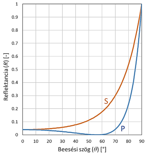
külső visszaverődés ( n'/n = 1.5 )
