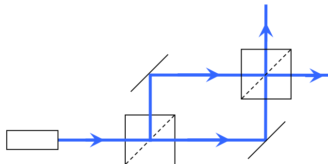
Mach-Zehnder
