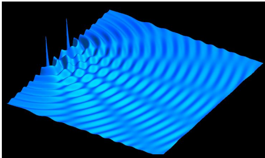
Két pontforrás (hullámkép pl. vízfelszínen)
