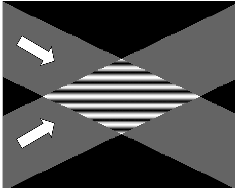
Két síkhullám interferenciája
