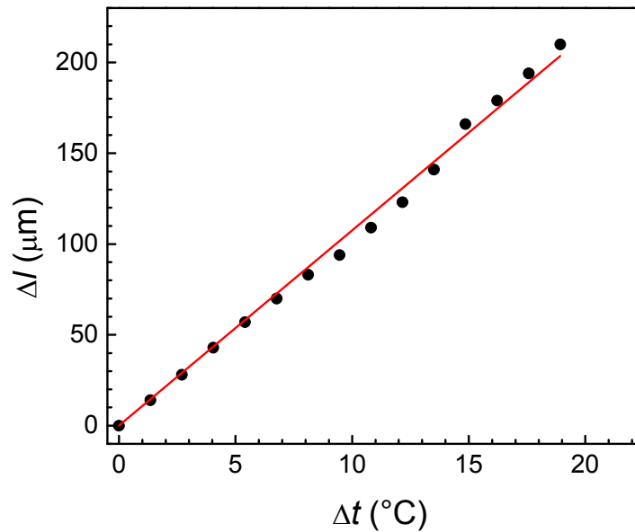
2. ábra. A mért megnyúlás értékek a referencia hőmérséklettől való eltérés függvényében. A folytonos vonal a mérési adatokra a legkisebb négyzetek módszerével illesztett, origón átmenő egyenest mutatja.
