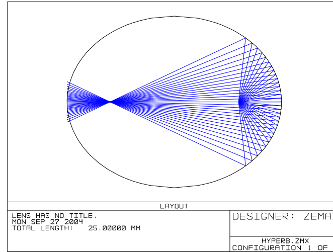
ellipszoid tükör
