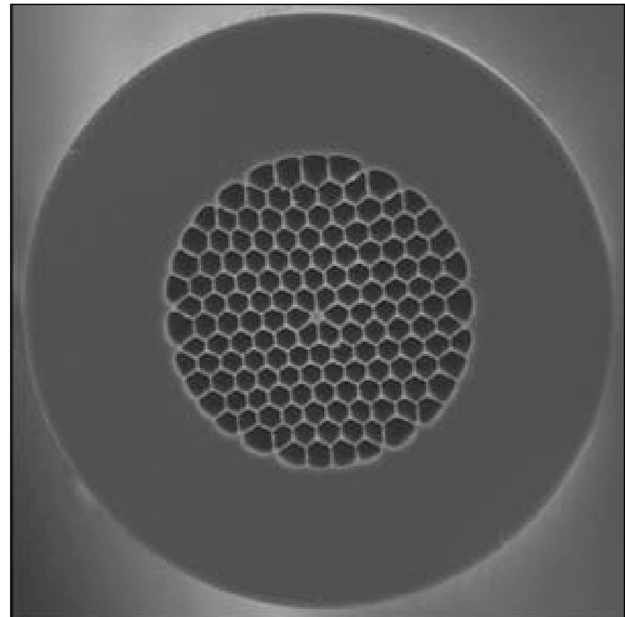
Fotonikai kristály
