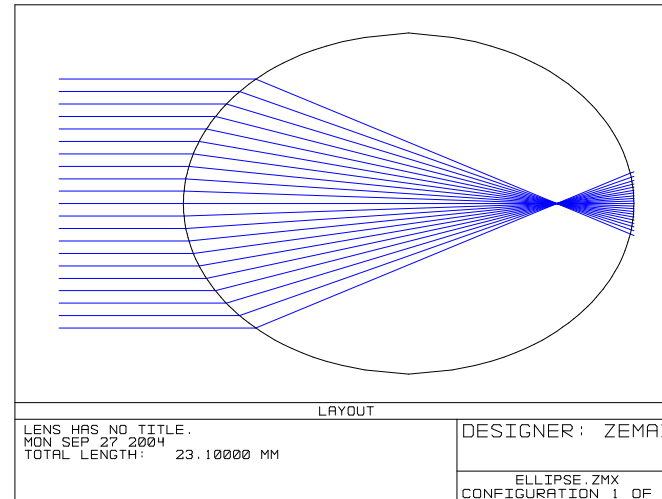
ellipszoid lencse
