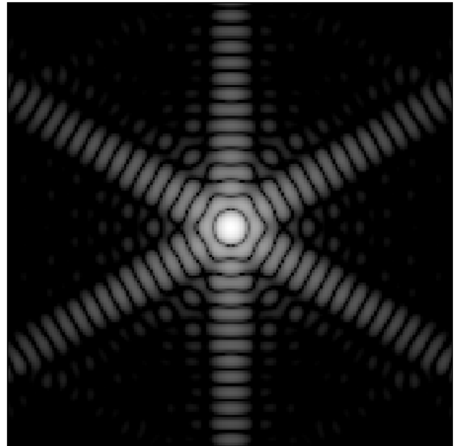
Fraunhofer-diffrakciós kép
