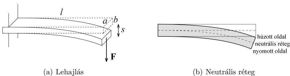
7.4. ábra. Rúd lehajlása
