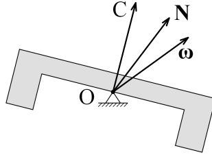
6.18. ábra. Egyensúlyából kibillentett erőmentes, szimmetrikus pörgettyű
